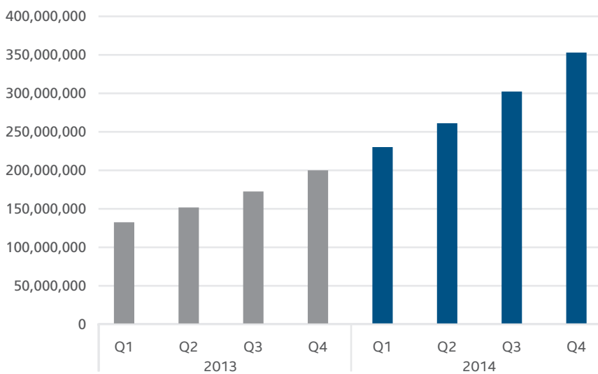
Total Malware
