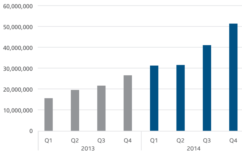
New Malware
